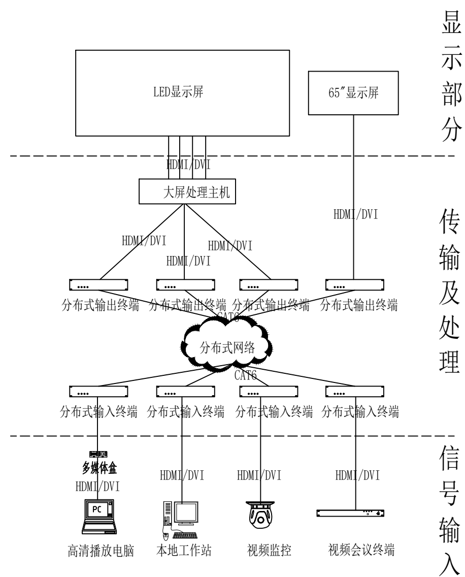
分布式系统图
