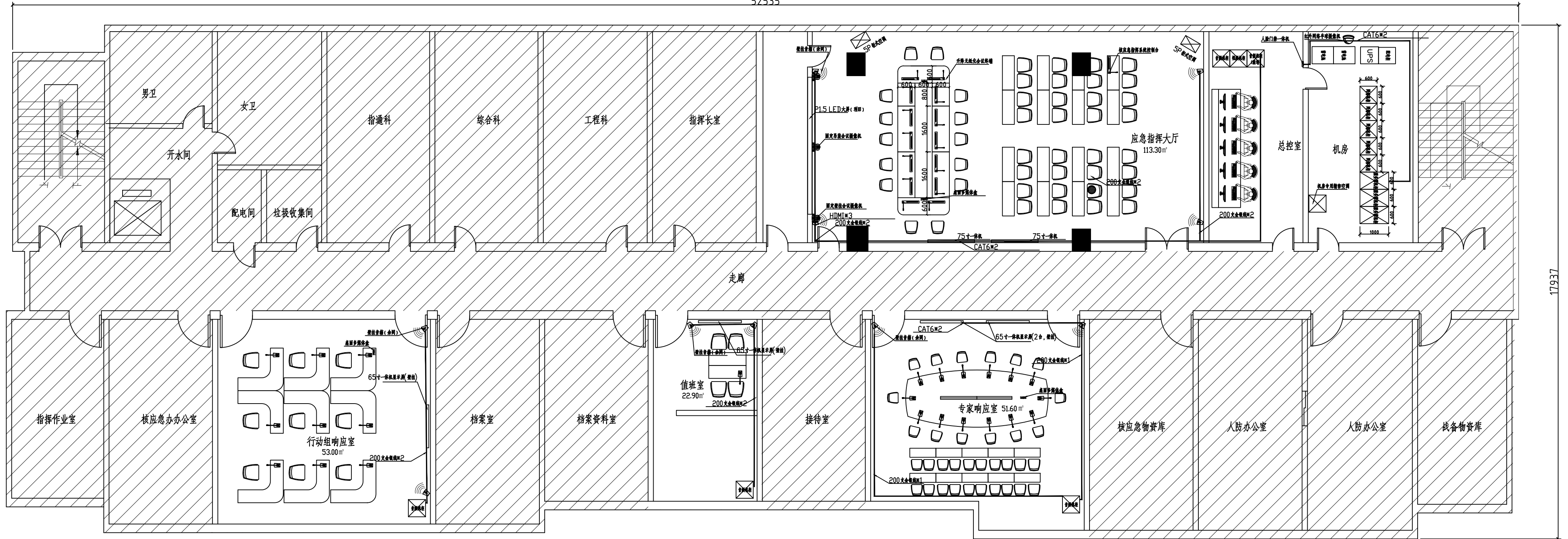
5楼天花弱电管线图
